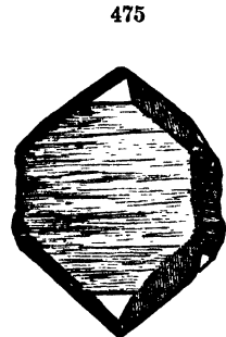
Haddam.
